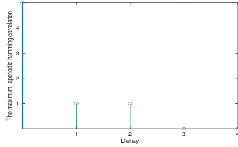
Fig. 1 The maximum aperiodic HC of \mathcal{S}
